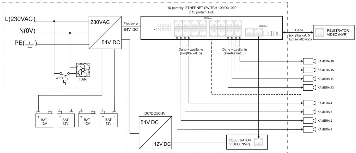
Rys. 1. Schemat blokowy.
